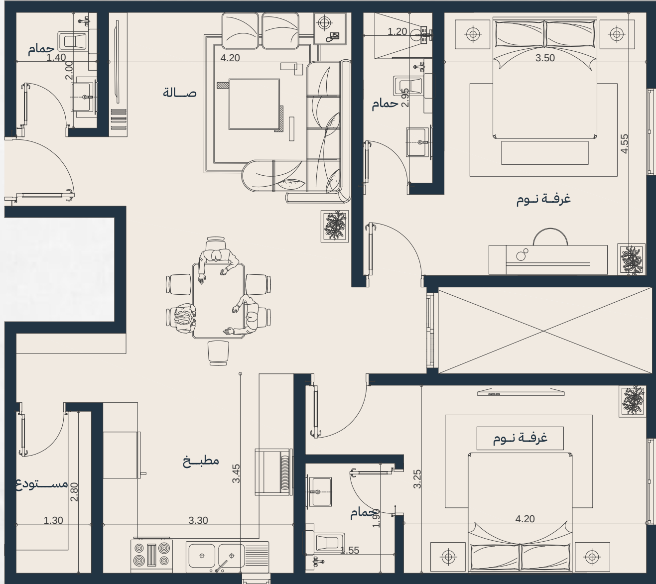
مخطط الشقة
